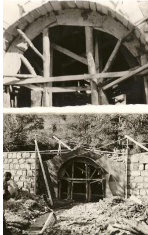
Ponte in muratura strada forestale
